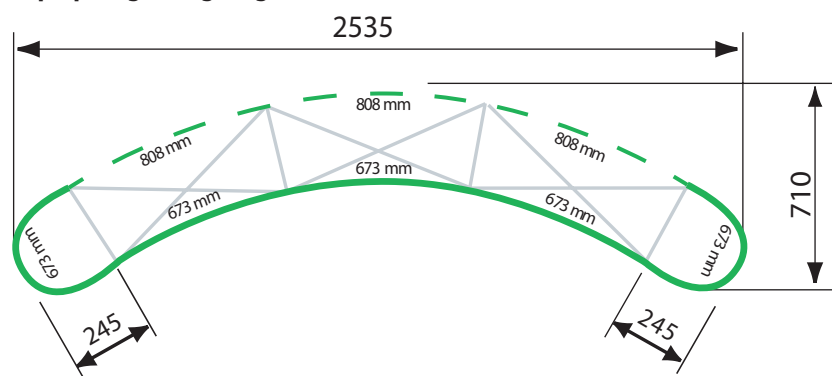
Pop Up Magnetic gebogen, 3 x 3 Felder
