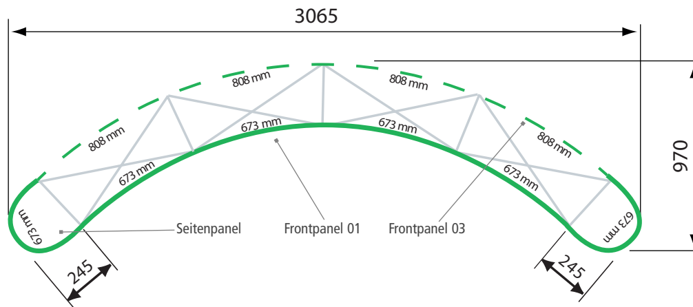
Pop Up Magnetic gebogen, 4 x 3 Felder
